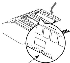
内存模块中的槽口
