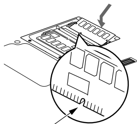
模块内槽口
