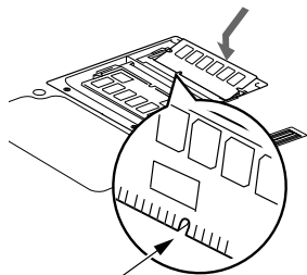
記憶體模塊中的槽口
