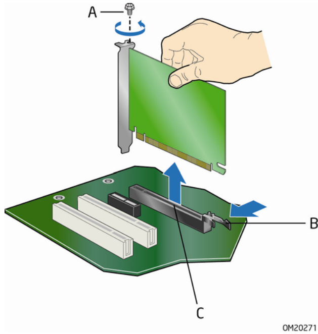
图 17. 拆卸 PCI Express x16 卡
