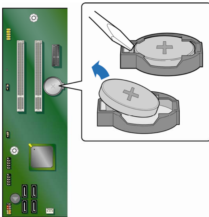
图 26. 拆卸电池
