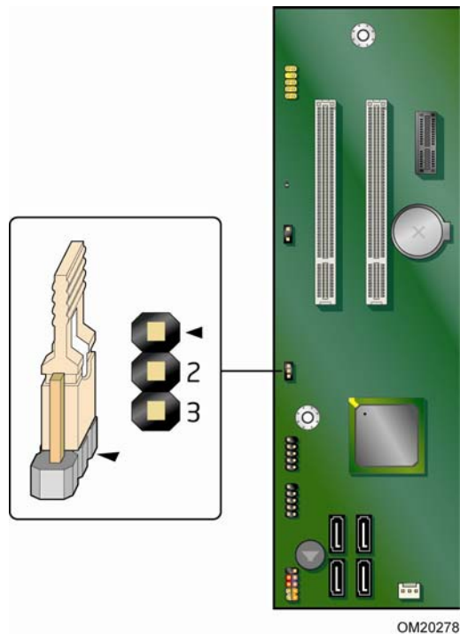
图 25. BIOS 配置跳线块位置
