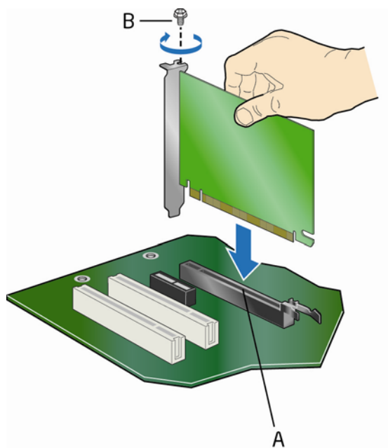
图 16. 安装 PCI Express x16 卡
