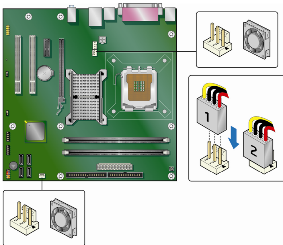
图 22. 机箱风扇接头连接器位置
