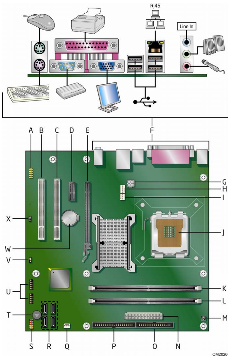
图 1. 台式机主板 D945GCNL 组件
