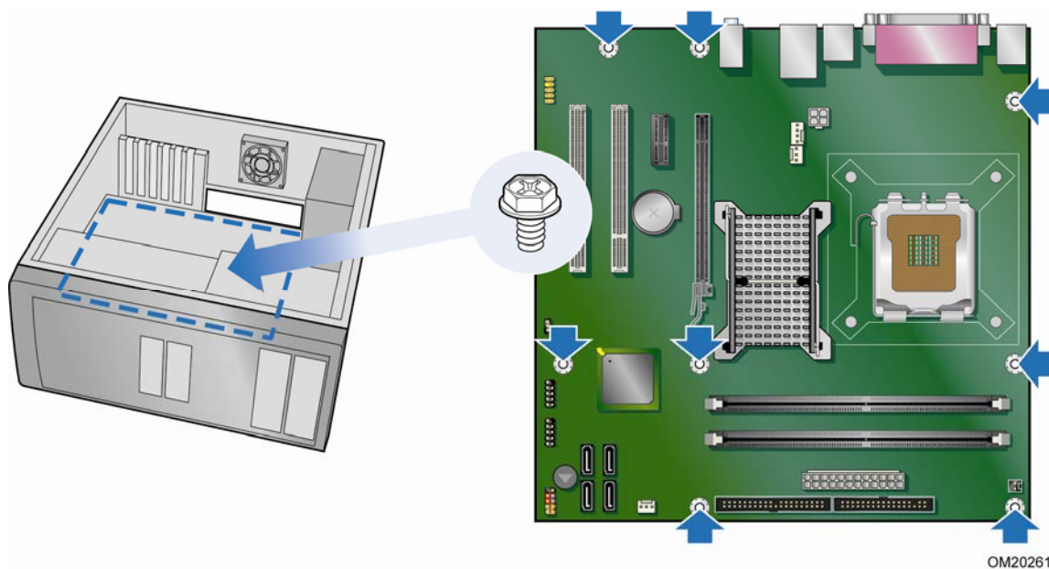
图 5. 台式机主板 D945GCNL 安装螺丝孔位置
