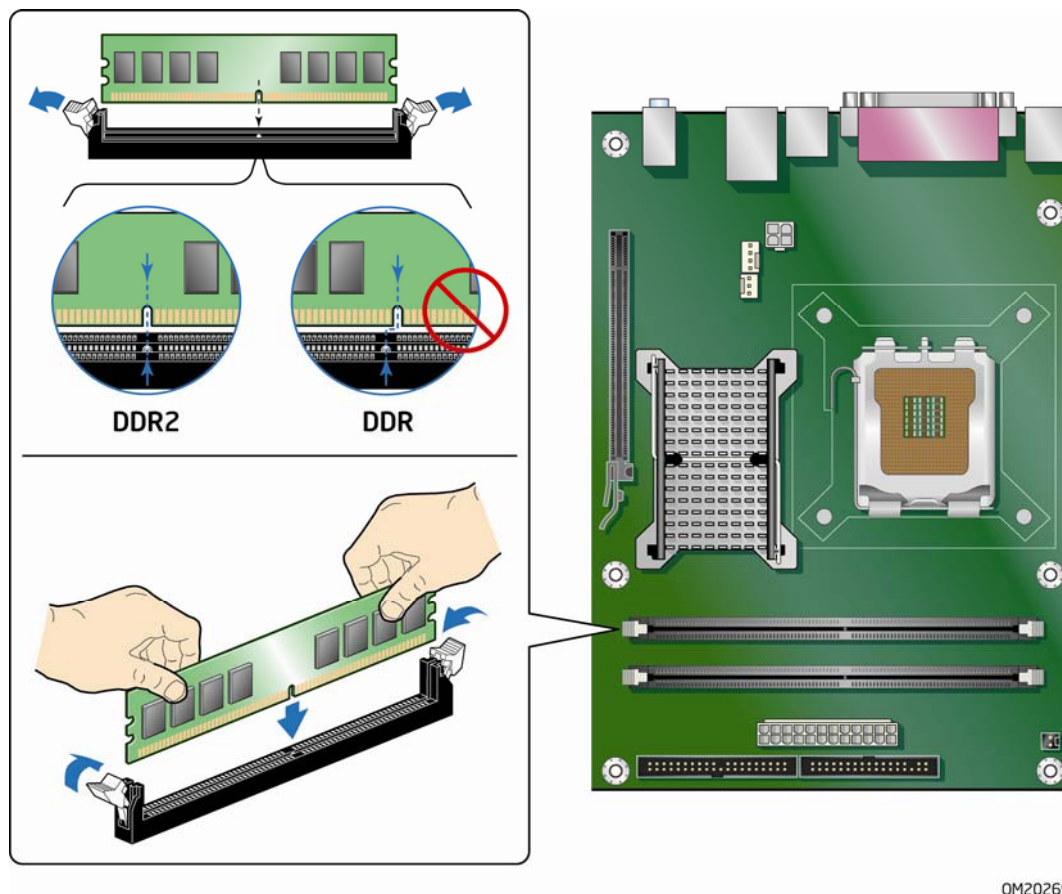
图 15. 安装 DIMM
