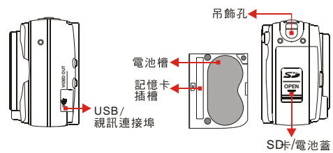
側部圖示
