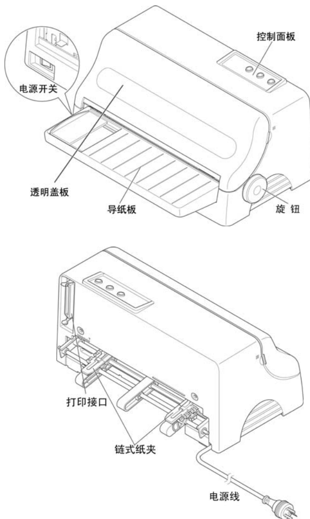
打印机部件名称示意图
