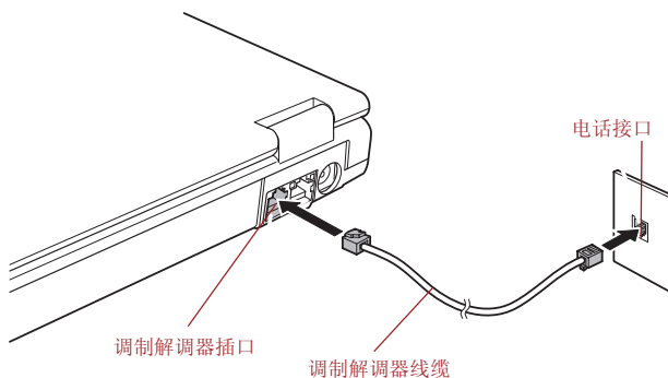
图 4-12 连接内置调制解调器
