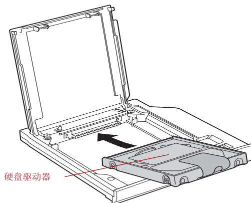
图8-15 插入硬盘驱动器
