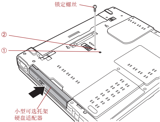
图 4-5 插入小型可选托架硬盘适配器
