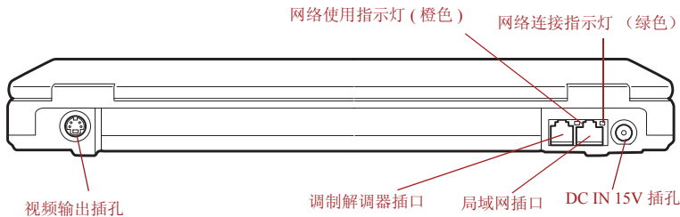
图 2-4 电脑的后侧
