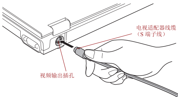
图 8-18 将 S-Video 线缆连接至视频输出插孔
