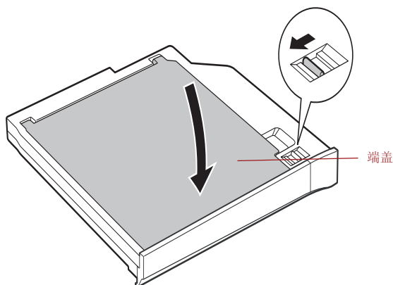
图8-16 合上端盖
