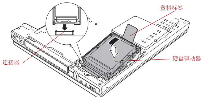
图 8-13 安装硬盘驱动器
