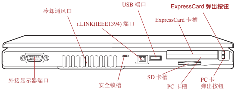
图 2-2 电脑的左侧
