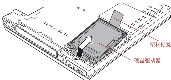
图 8-12 取出硬盘驱动器
