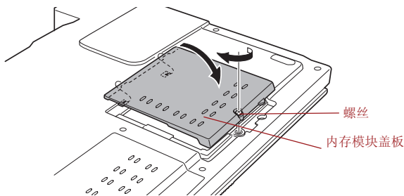
图 8-9 合上内存模块插槽盖板
