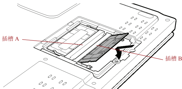
图 8-8 放置内存模块
