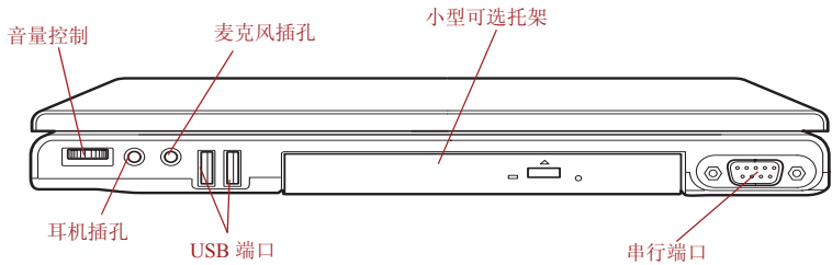
图 2-3 电脑的右侧
