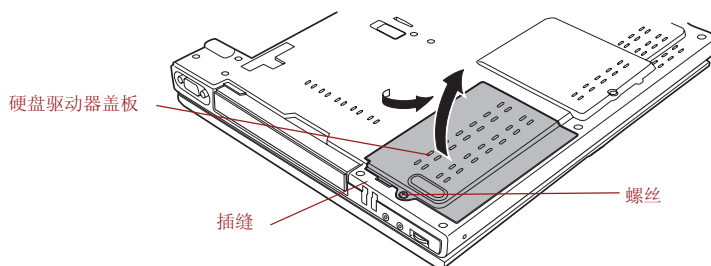
图 8-11 取出硬盘驱动器盖板
