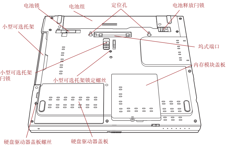
图 2-5 电脑的底部
