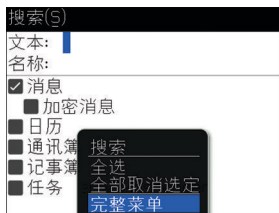
图 12. 快捷菜单
