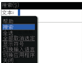
图 11. 完整菜单
