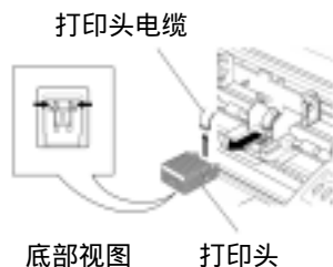
图 A-2 更换打印头
