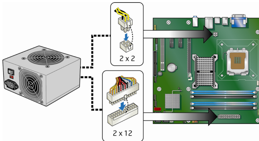
图 27. 连接电源系统电缆
