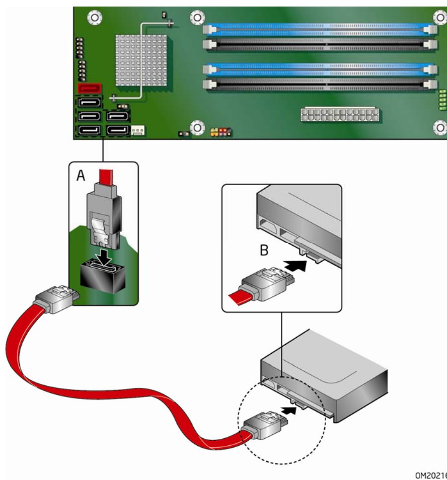
图 22. 连接串行 ATA 电缆
