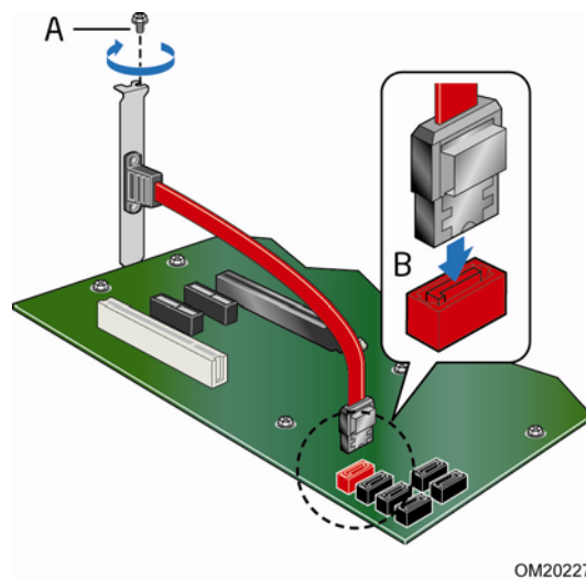
图 23. 连接外置串行 ATA 适配器固定架
