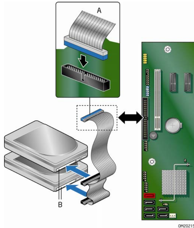
图 21. 连接 IDE 电缆
