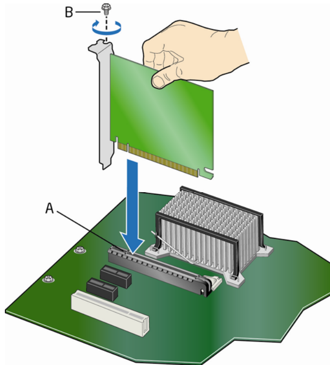
图 19. 安装 PCI Express x16 卡
