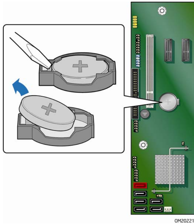
图 29. 拆卸电池
