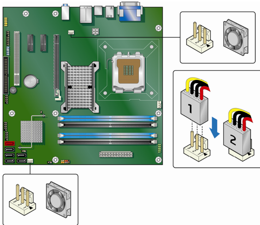
图 26. 机箱风扇接头连接器位置
