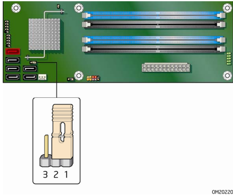
图 28. BIOS 配置跳线块位置
