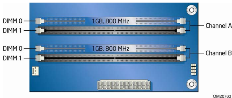
图 13. 两条 DIMM 双通道内存配置
