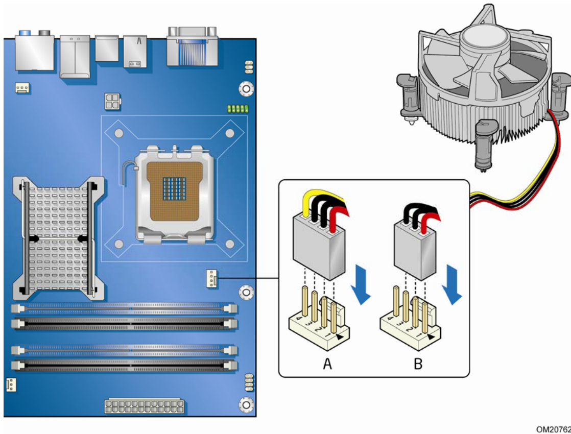
图 12. 连接处理器风扇散热器电缆
