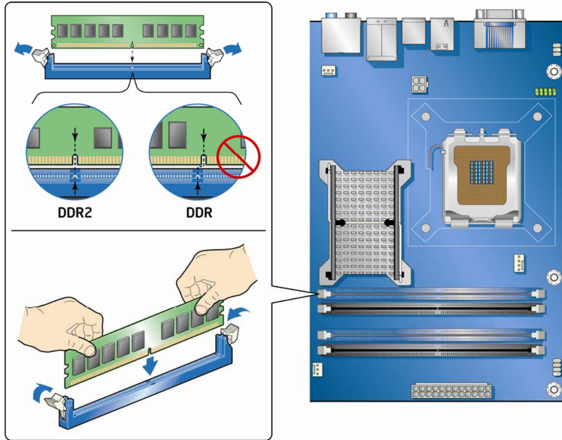
图 17. 安装 DIMM
