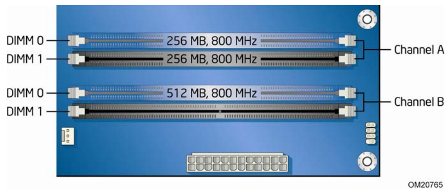
图 15. 三条 DIMM 双通道内存配置
