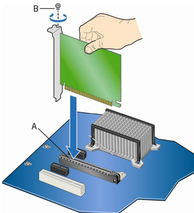
图 18. 安装 PCI Express x16 卡
