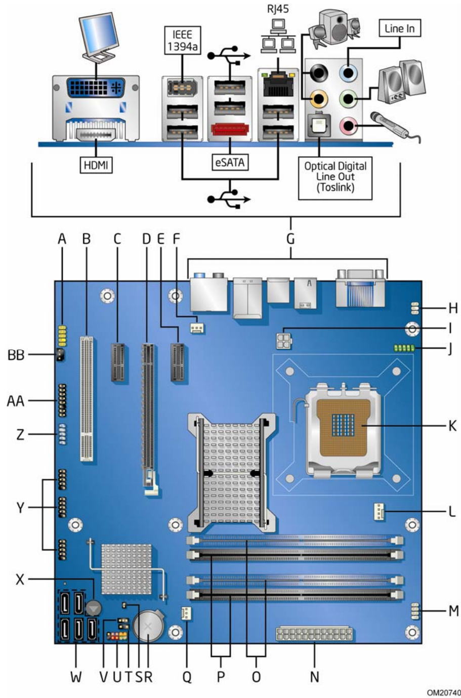
图 1. 台式机主板 DG45ID 组件
