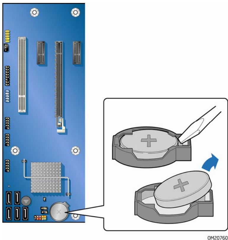
图 26. 拆卸电池
