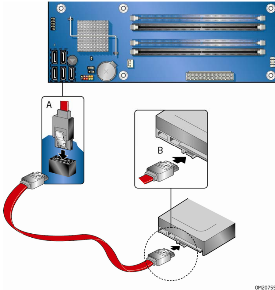
图 20. 连接串行 ATA 电缆
