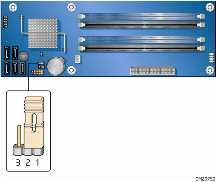
图 25. BIOS 配置跳线块位置
