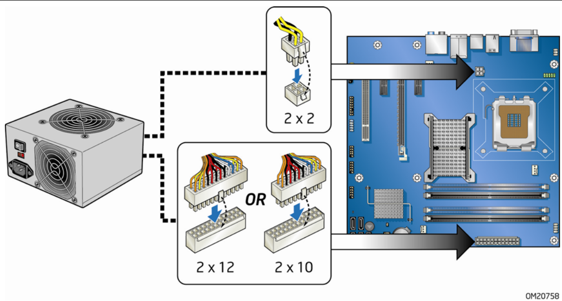
图 24. 连接电源系统电缆
