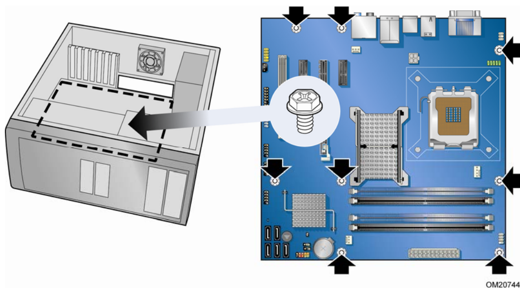
图 5. 台式机主板 DG45ID 安装螺丝孔位置
