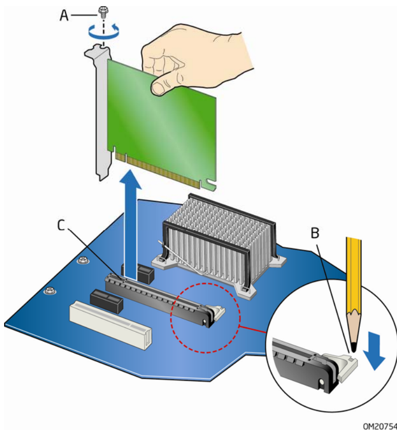
图 19. 拆卸 PCI Express x16 卡
