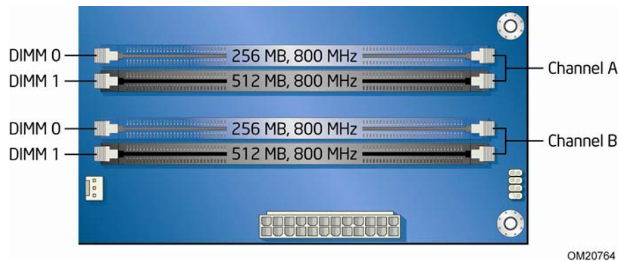
图 14. 四条 DIMM 双通道内存配置
