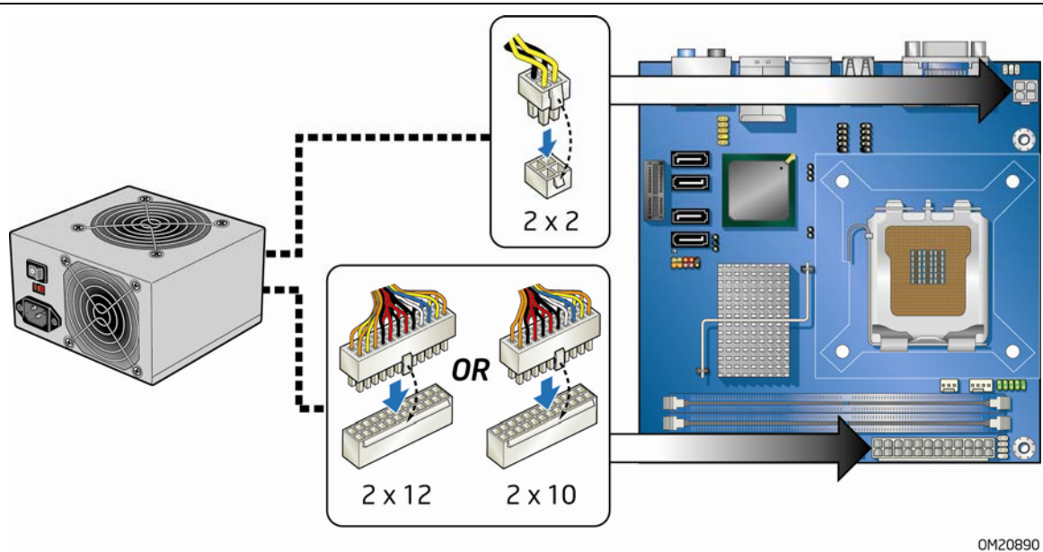
图 20. 连接电源系统电缆
