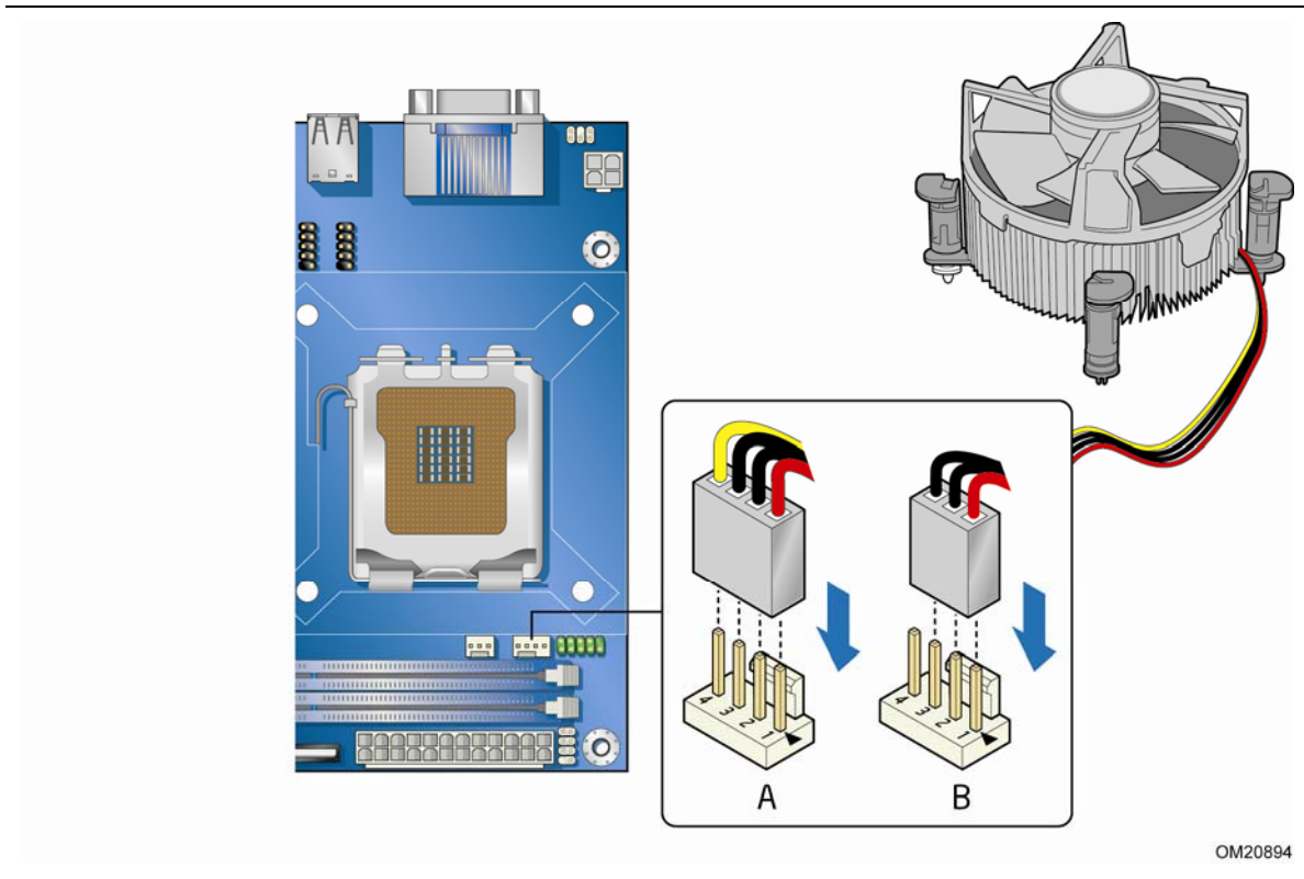
图 12. 连接处理器风扇散热器电缆
