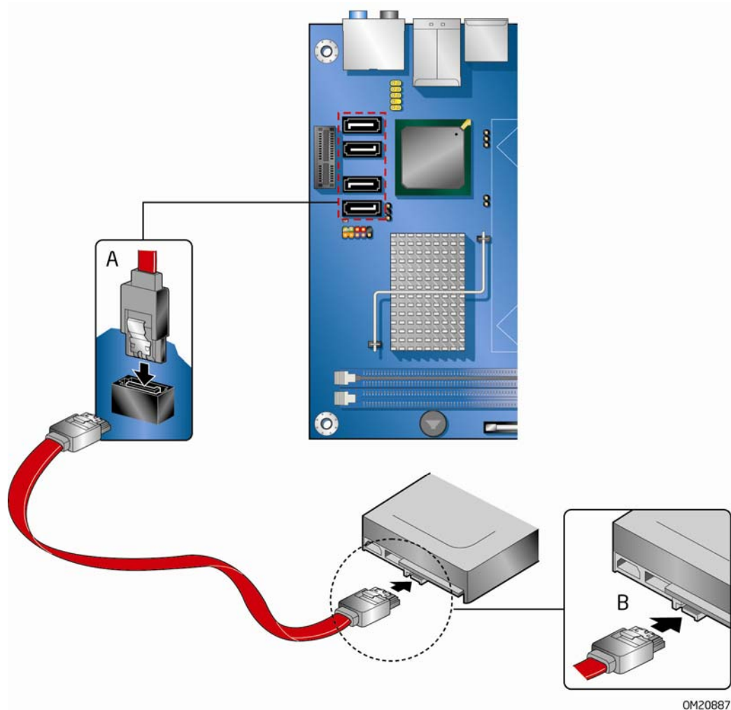
图 16. 连接串行 ATA 电缆
