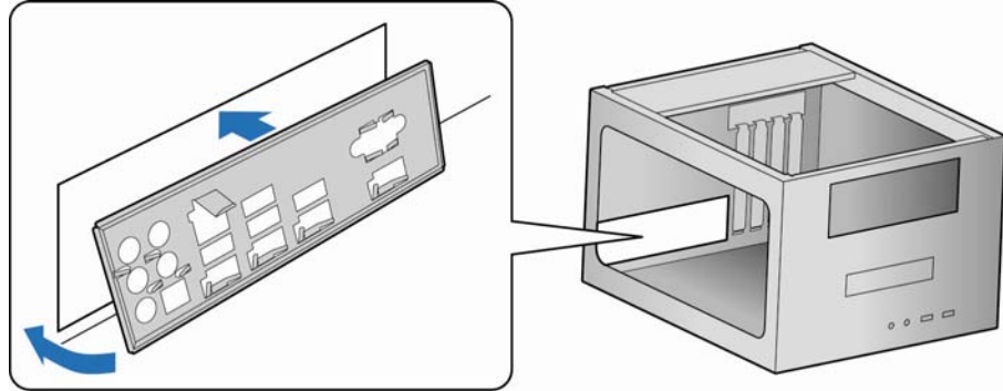
图 4. 安装 I/O 防护板
