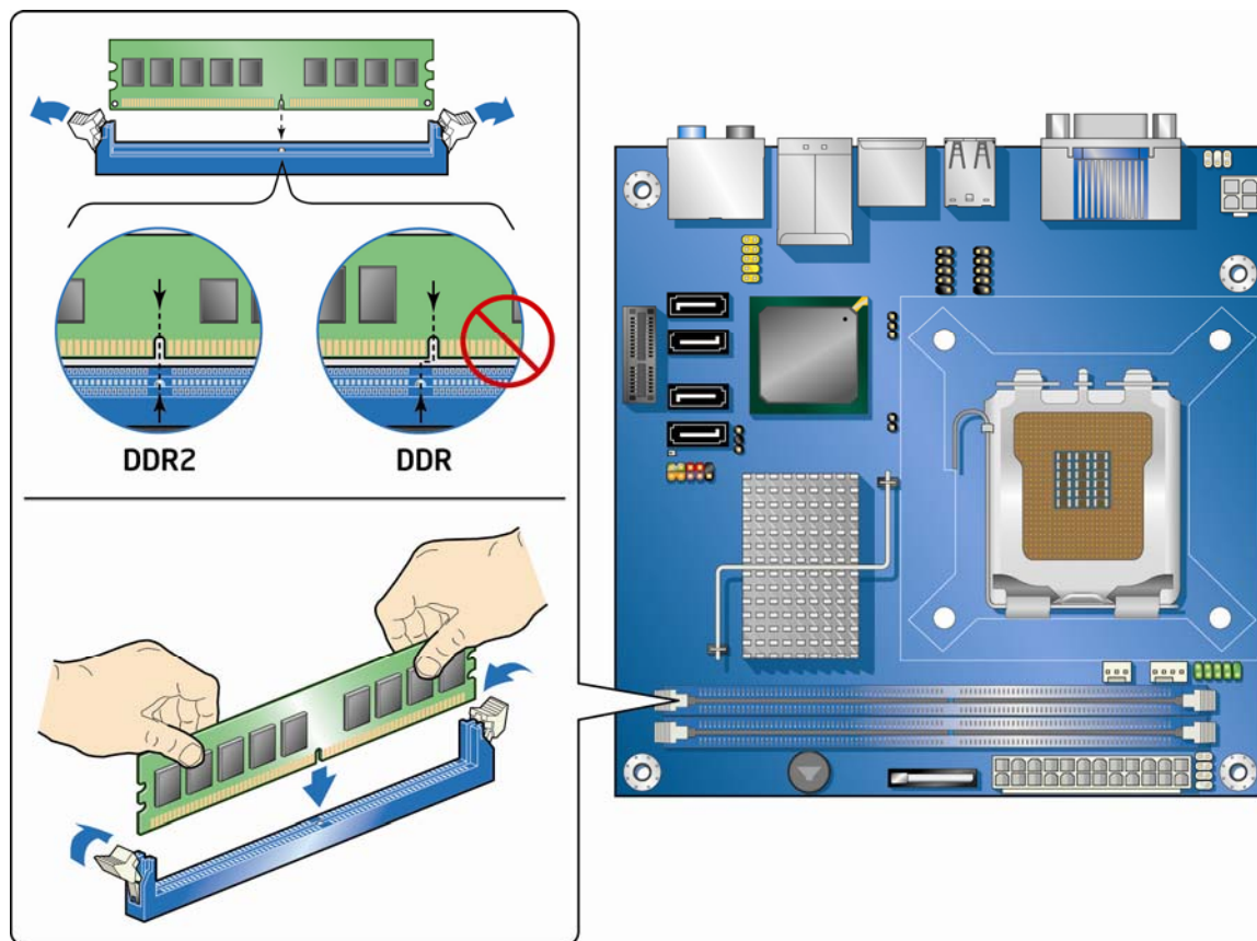
图 15. 安装 DIMM
