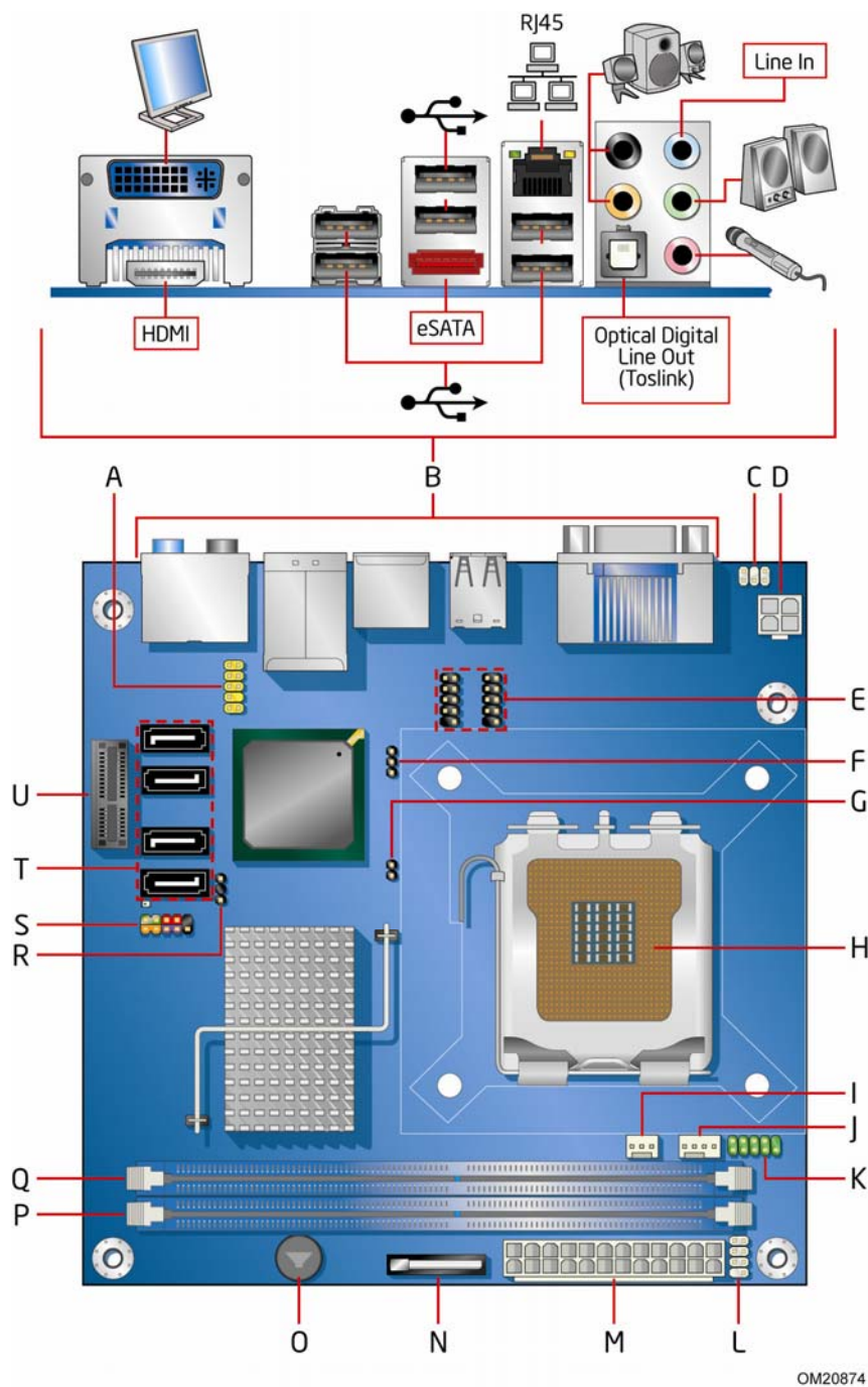
图 1. 台式机主板 DG45FC 组件
