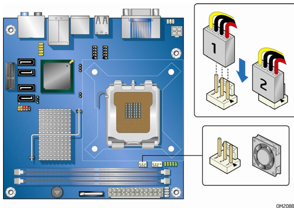
图 19. 机箱风扇接头连接器位置
