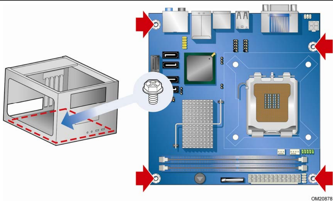
图 5. 台式机主板 DG45FC 安装螺丝孔位置
