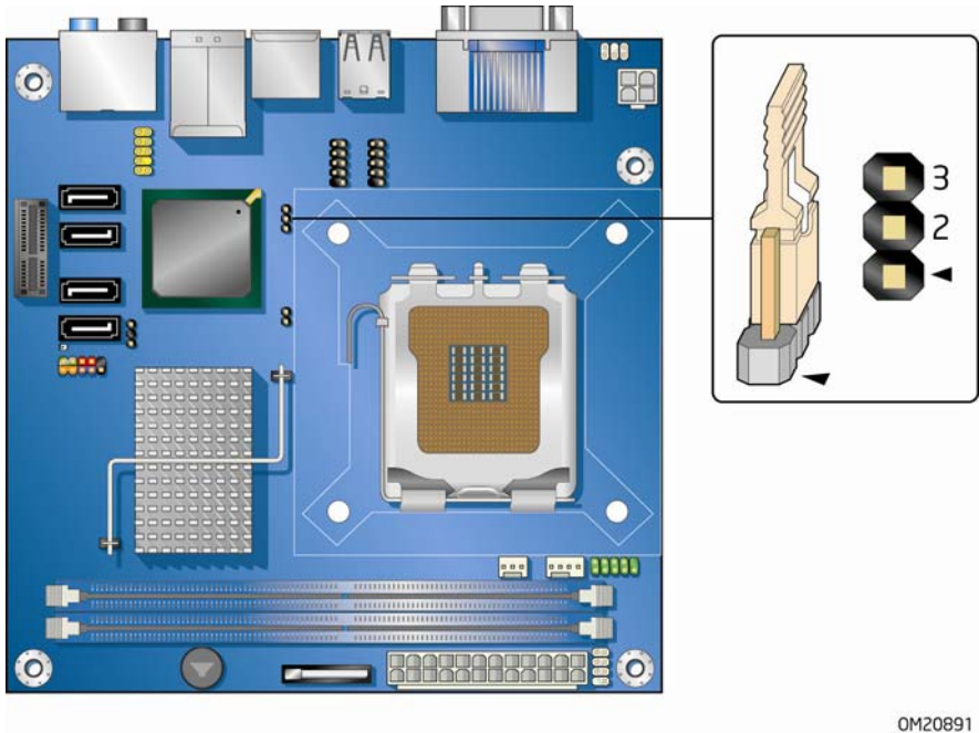
图 21. BIOS 配置跳线块位置
