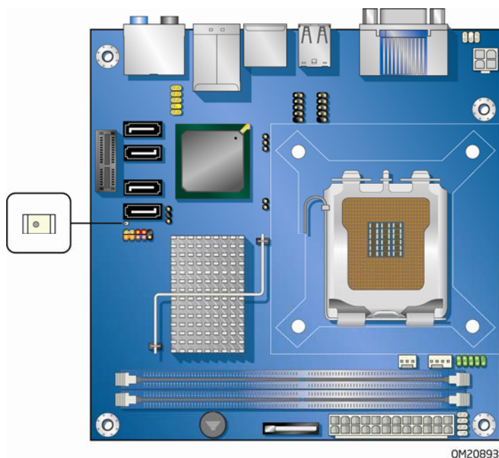
图 3. +5 V 备用电源指示灯位置
