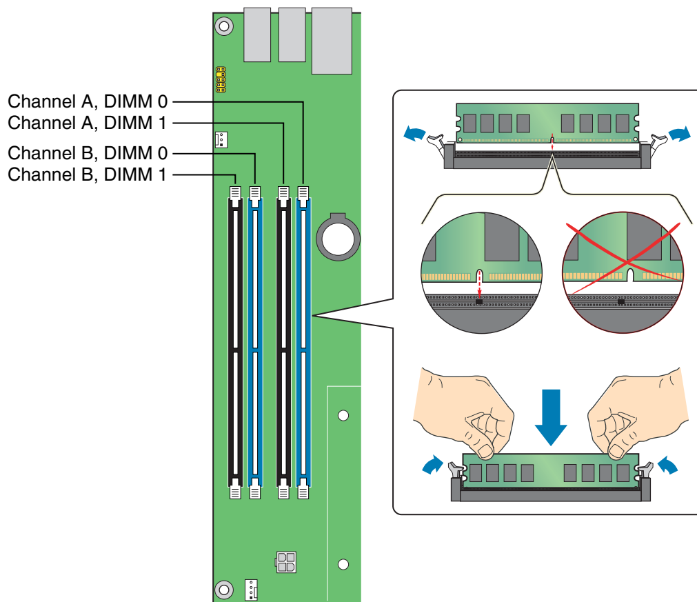
图 19. 安装 DIMM
