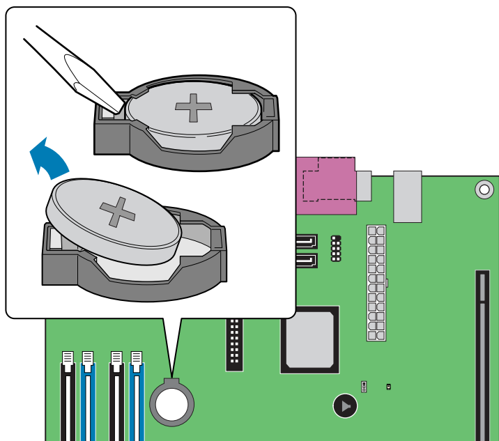
图 27. 拆卸电池
