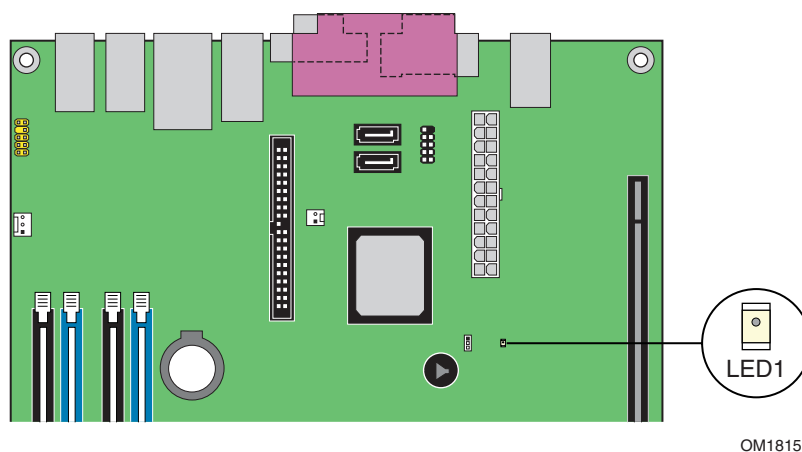
图 3. 备用电源指示灯位置
