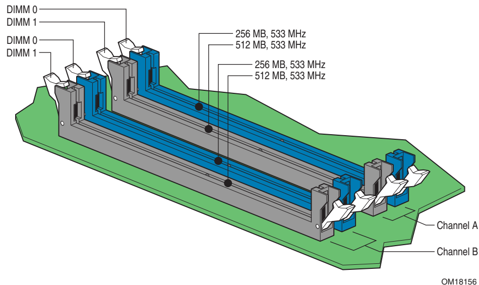
图 17. 双通道内存配置示例 2
