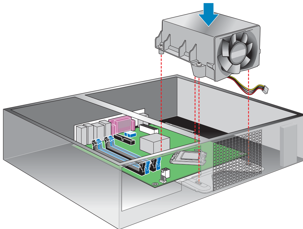
图 12. 将散热模块置于安装孔上方
