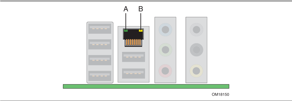
图 2. LAN 连接器 LED 指示灯
