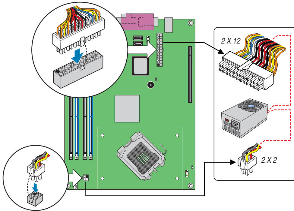
图 25. 连接电源系统电缆
