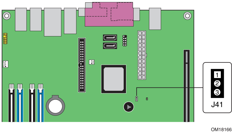
图 26. BIOS 配置跳线块位置
