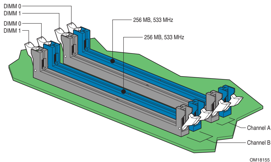
图 16. 双通道内存配置示例 1
