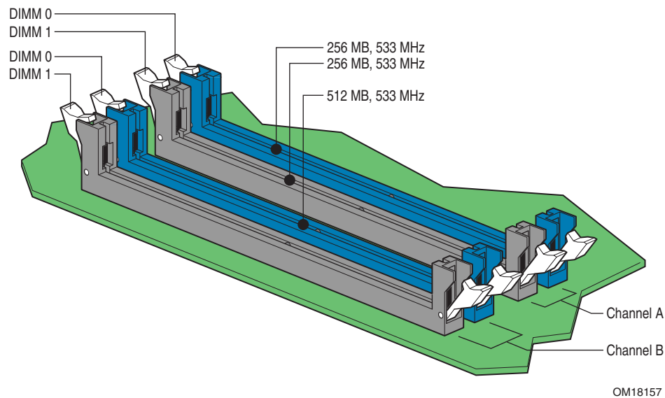
图 18. 双通道内存配置示例 3
