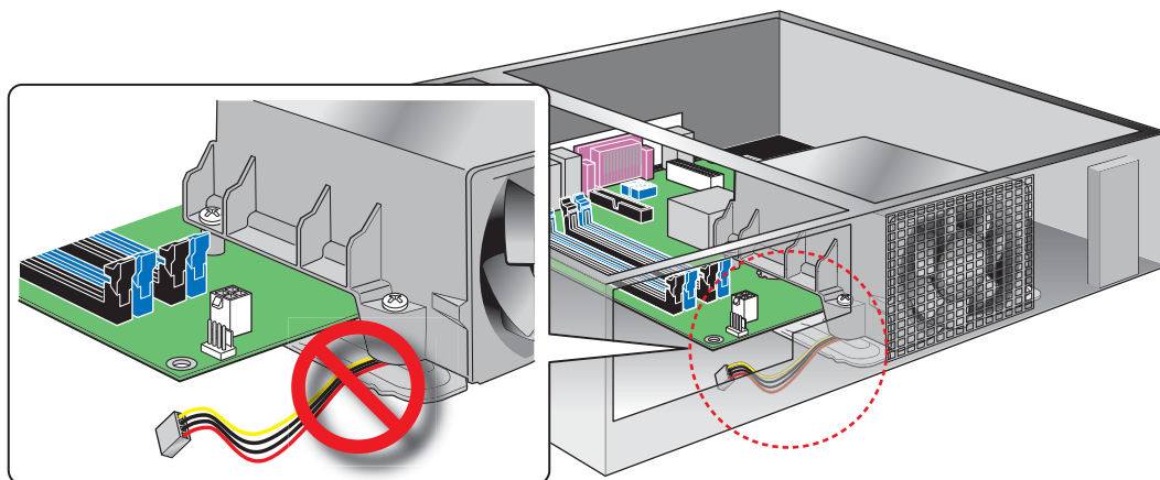
图 13. 注意不要压住散热模块风扇电缆
