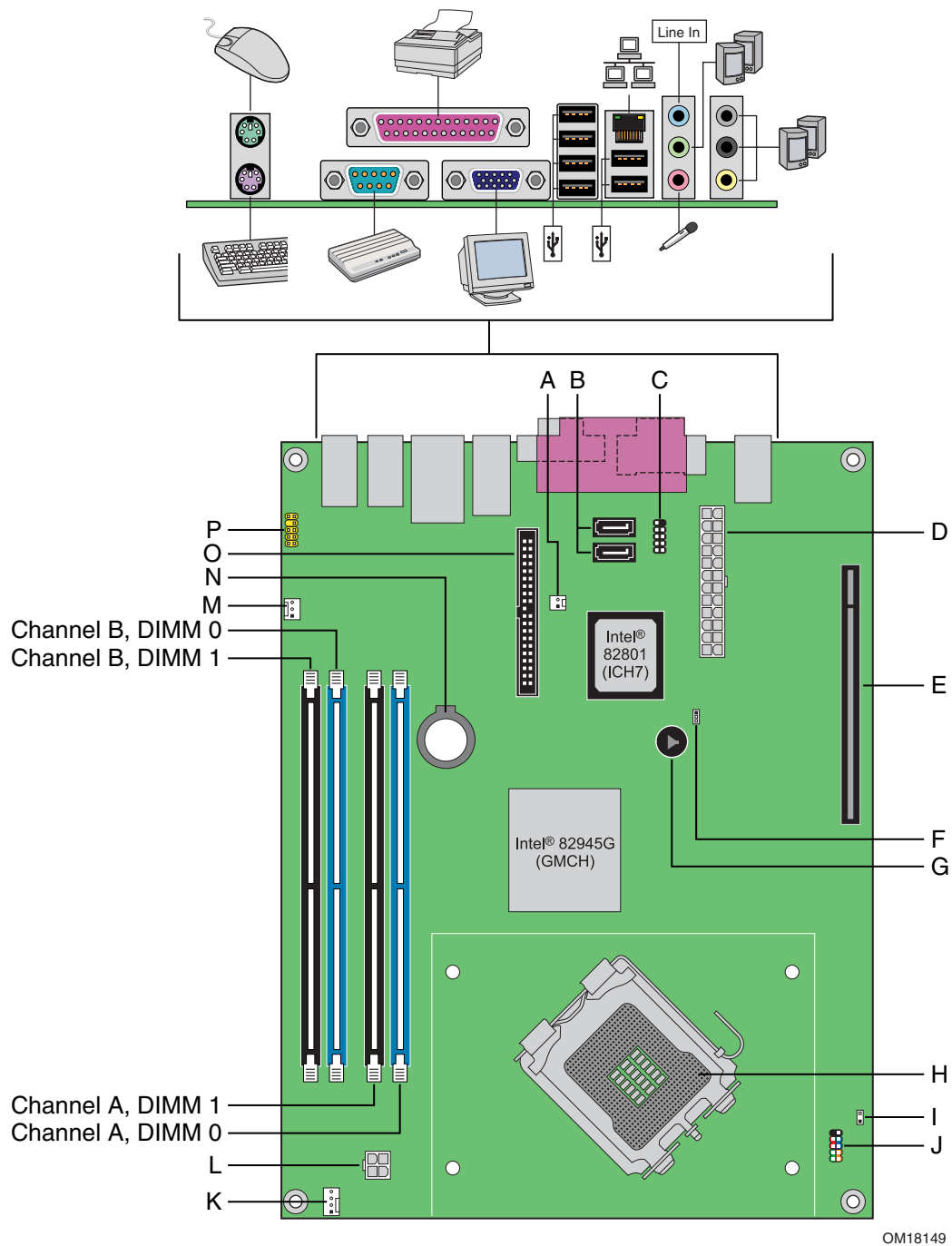
图 1. 台式机主板 D945GRW 组件
