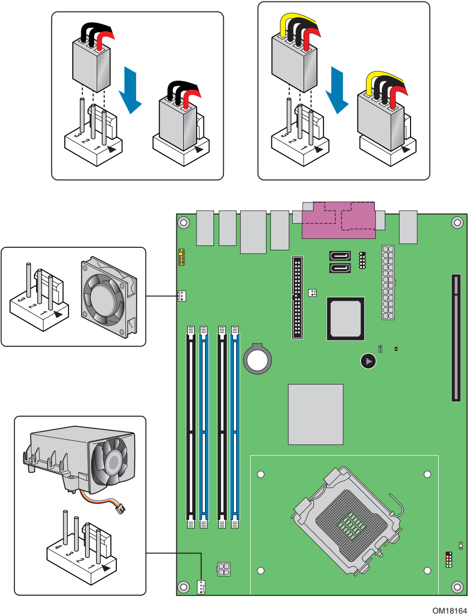
图 24. 风扇接头连接器位置
