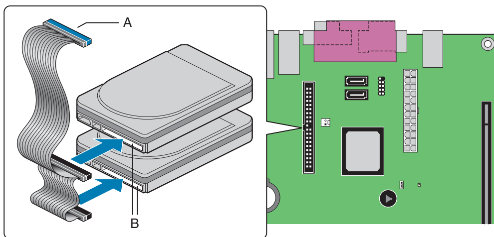
图 20. 连接 IDE 电缆
