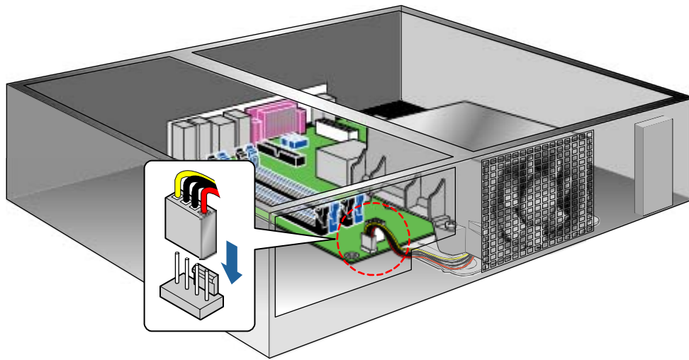
图 15. 连接散热模块风扇电缆
