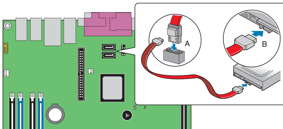
图 21. 连接串行 ATA 电缆
