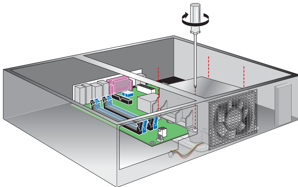
图 14. 固定散热模块
