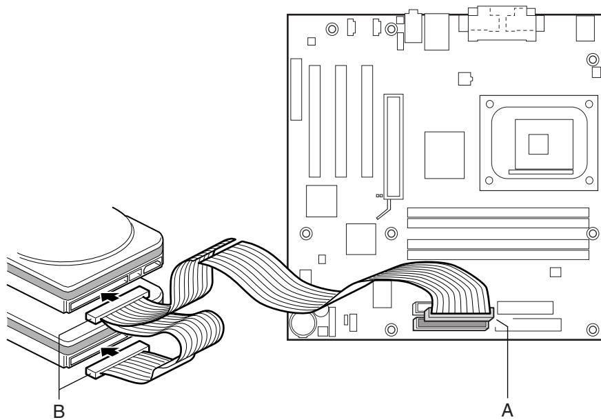
图 13. 连接 IDE 电缆
