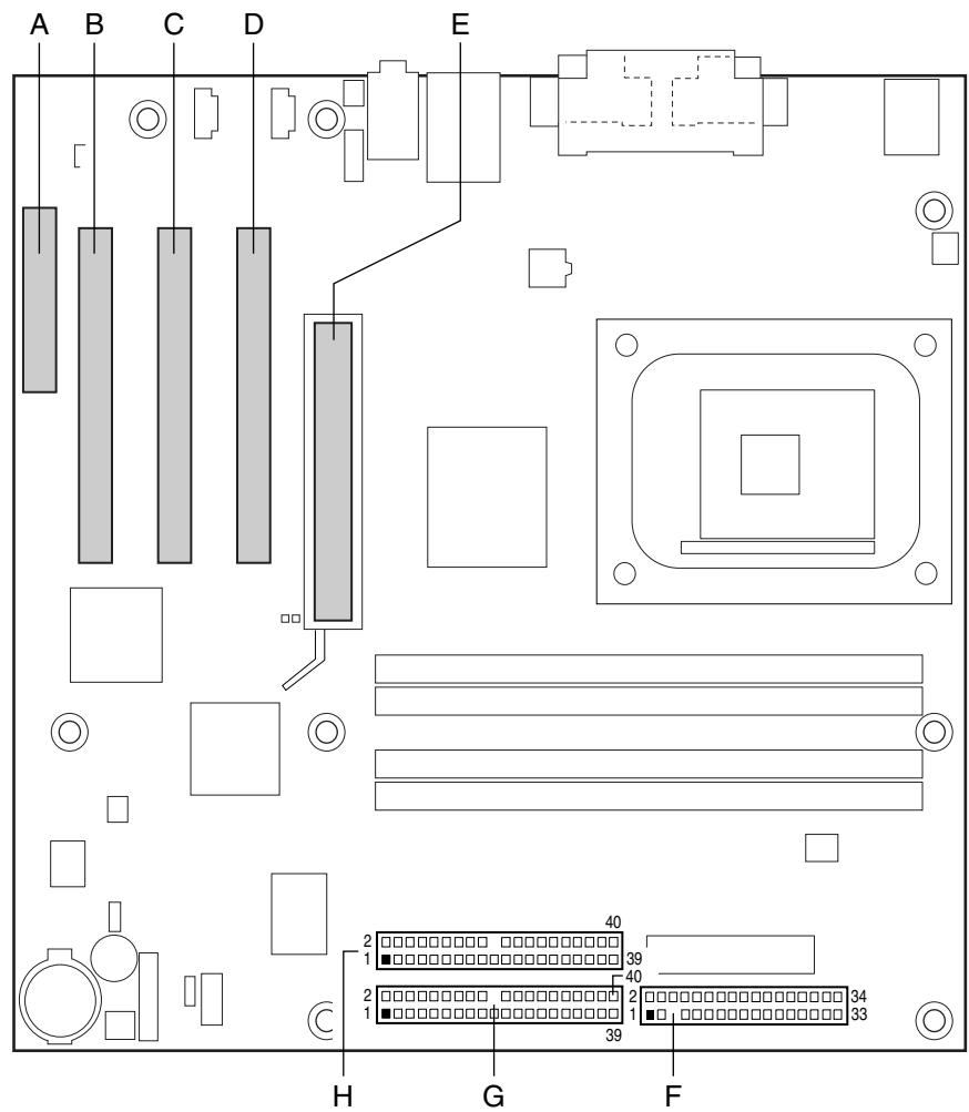
图 20 显示 D850EMD2 桌面母板上附加卡和外围设备接口连接器。
