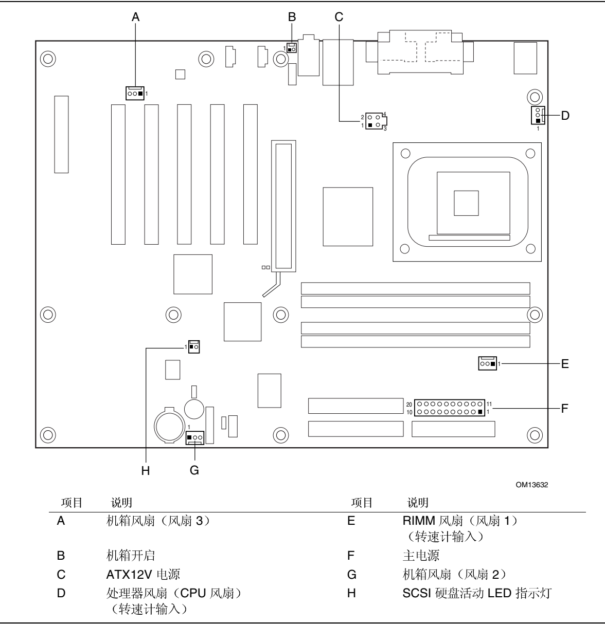
图 19. 桌面母板 D850EMV2 电源和硬件控制连接器
