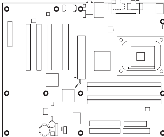
图 6. D850EMV2 桌面母板安装螺丝孔位
