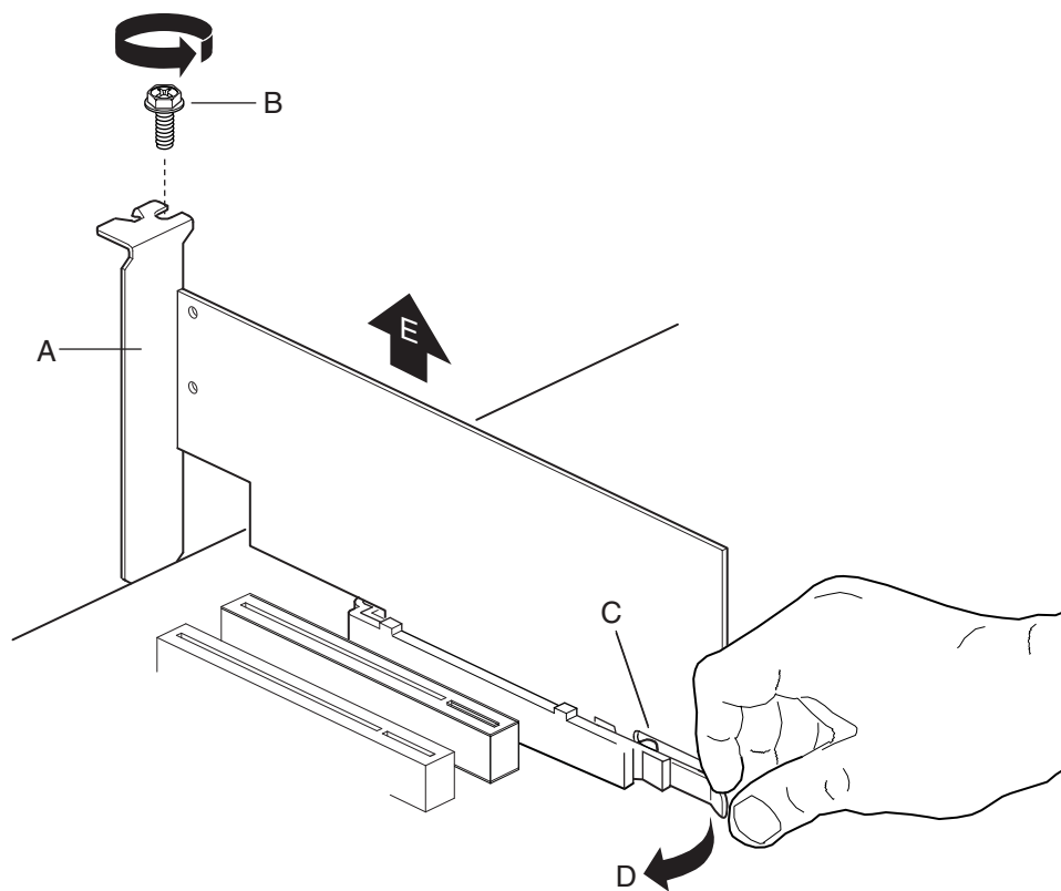
图 12. 拆卸 AGP 卡
