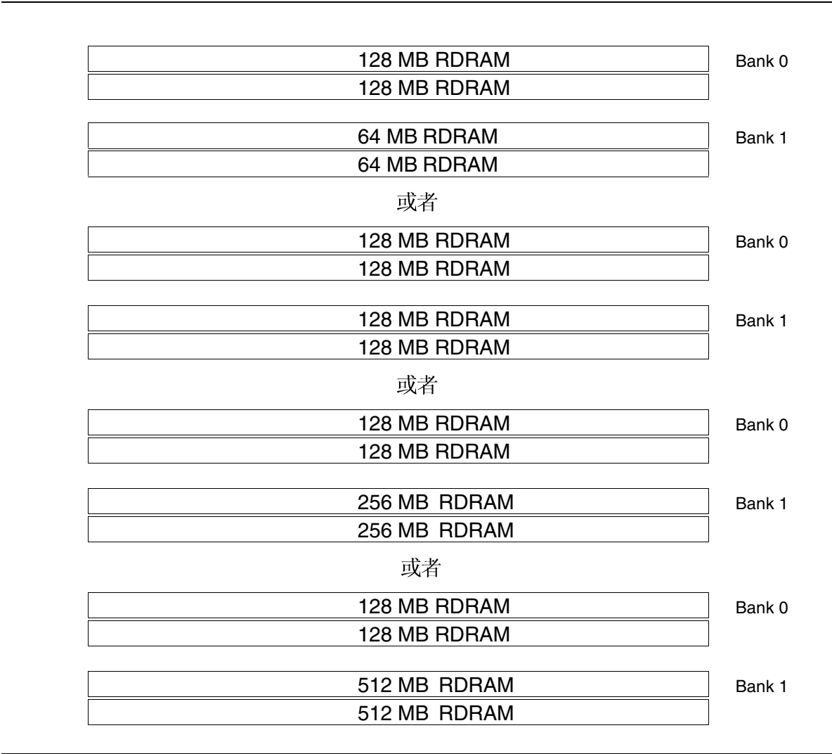
图 10. 安装 RIMM
