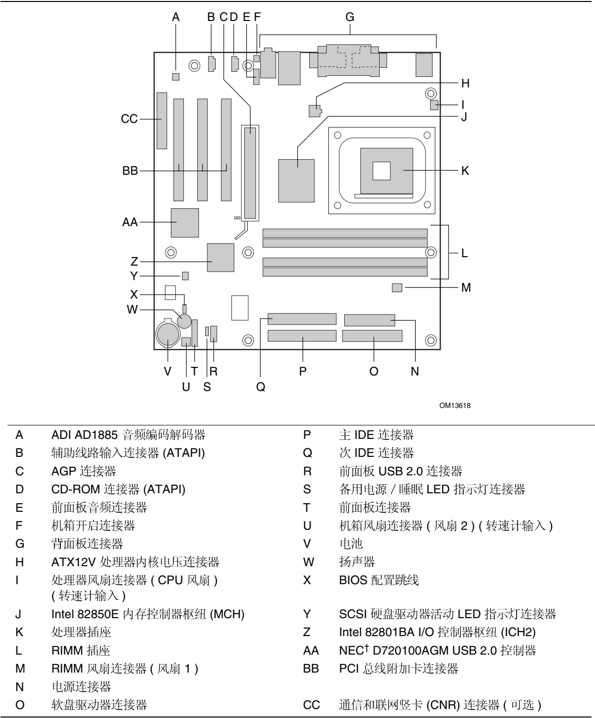
图 1. 桌面主板 D850EMD2 元件
