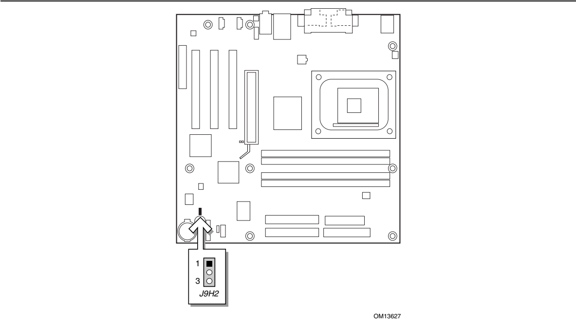
图 14. BIOS 配置跳线的位置
