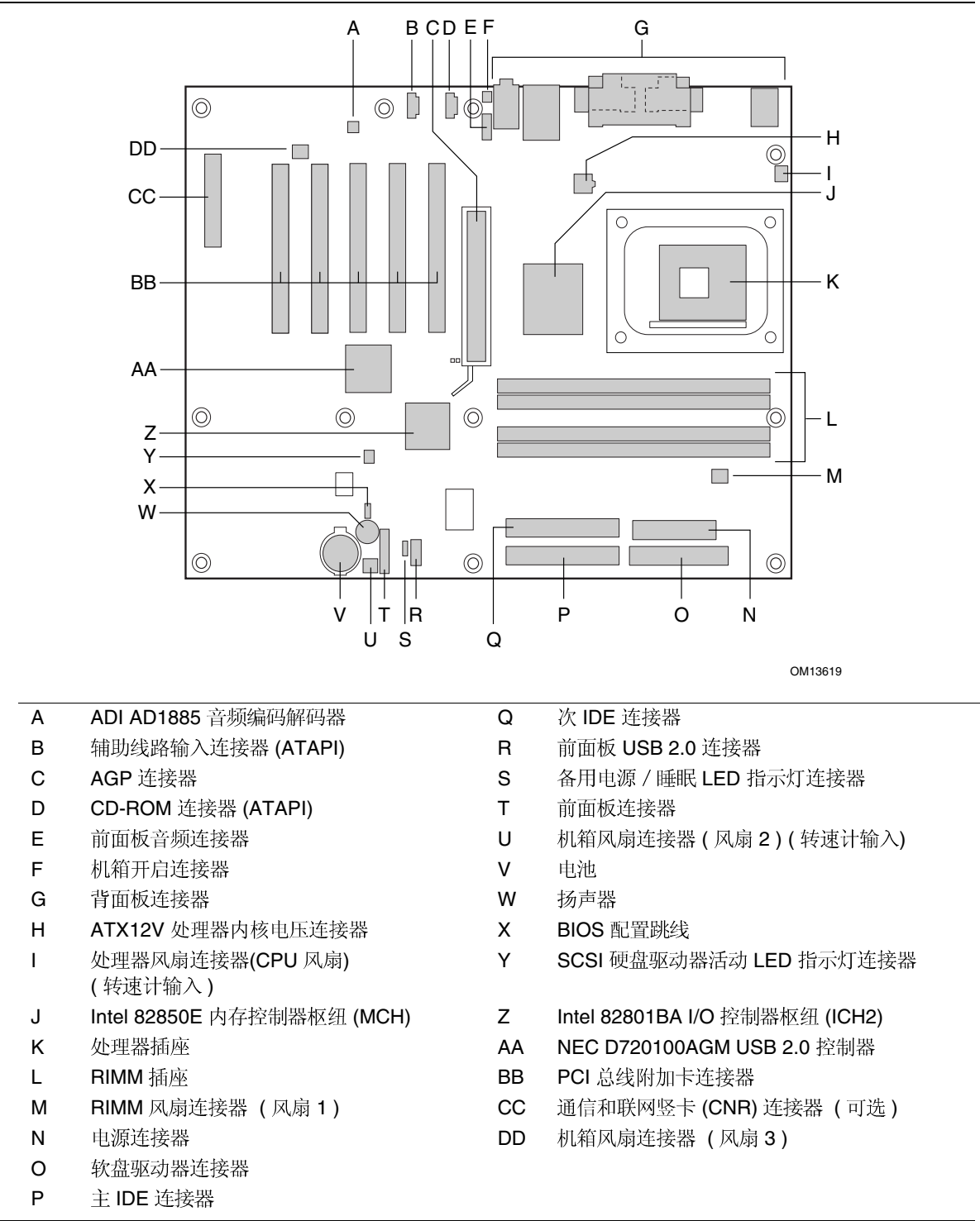
图 2. 桌面主板 D850EMV2 元件
