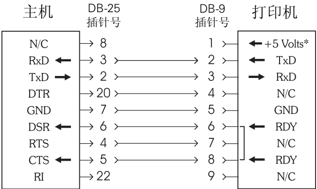
DB-25 插孔与 DB-9 插头
