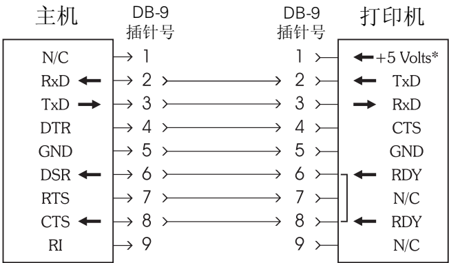
DB-9 插孔与 DB-9 插头
