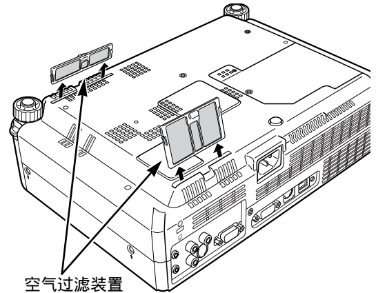
空气过滤装置 拔出并取下。
